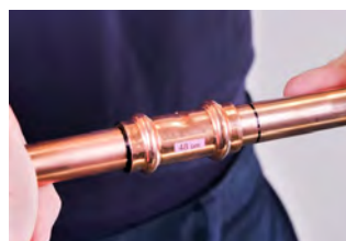
5. Inserción del tubo en el accesorio 5. Encaixar o tubo no acessório
