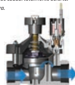
Vista transversal de una válvula PEB
